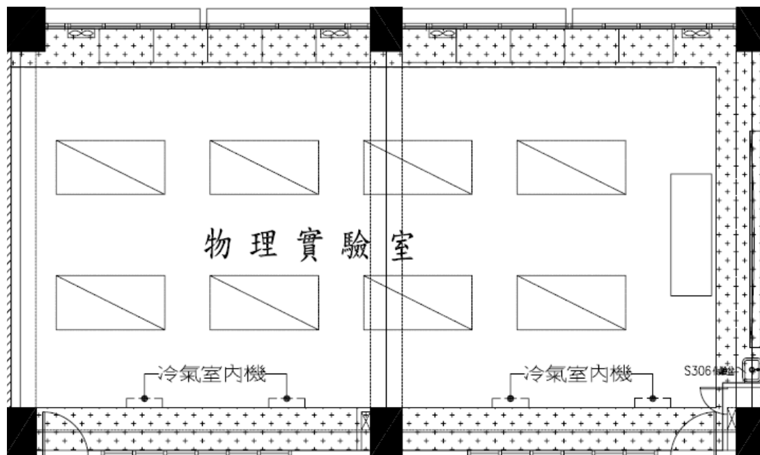
平面圖
