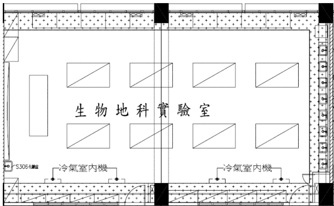
平面圖
