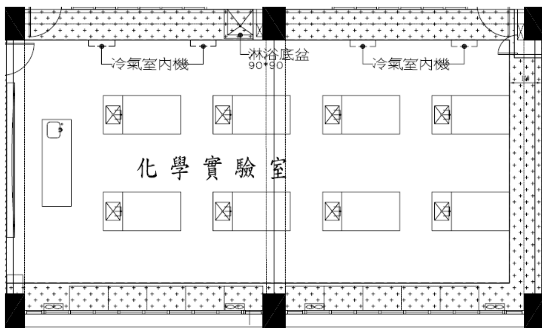
平面圖
