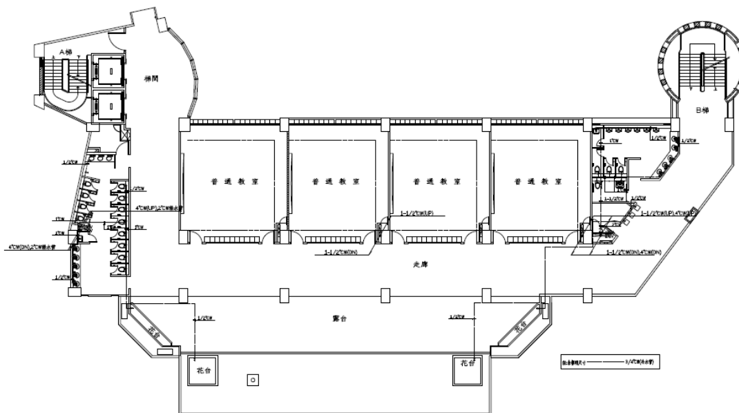
六層平面圖
