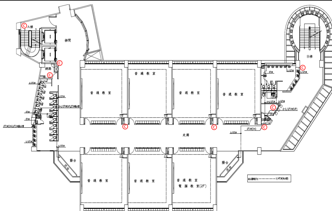
二層平面圖
