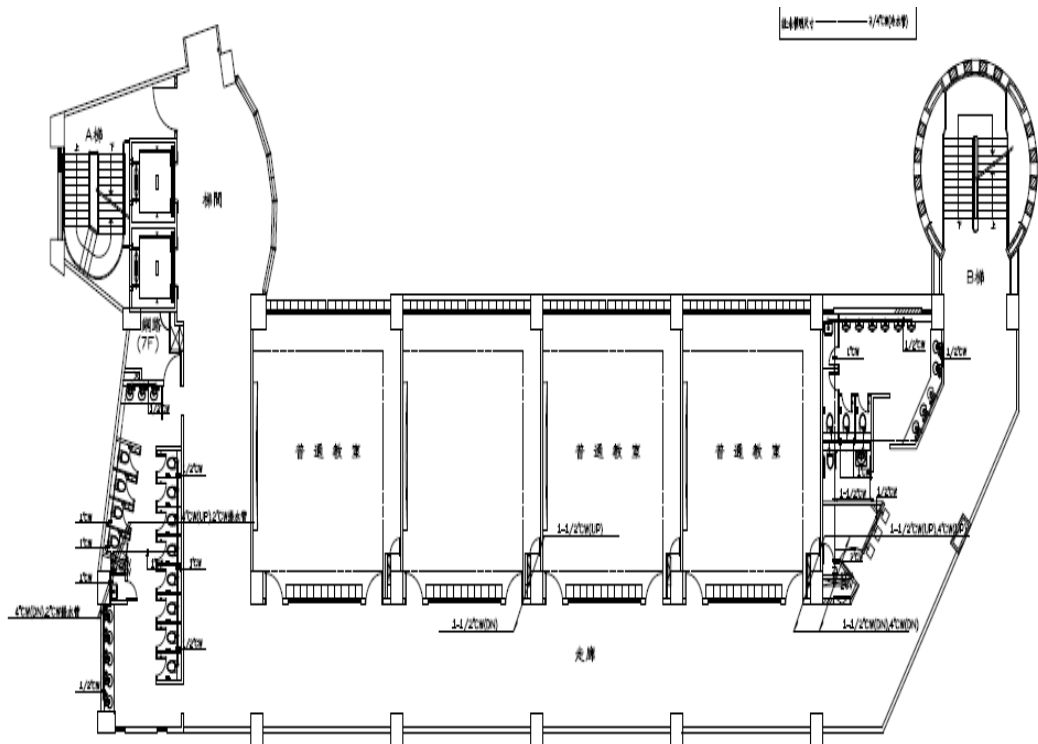
七層平面圖
